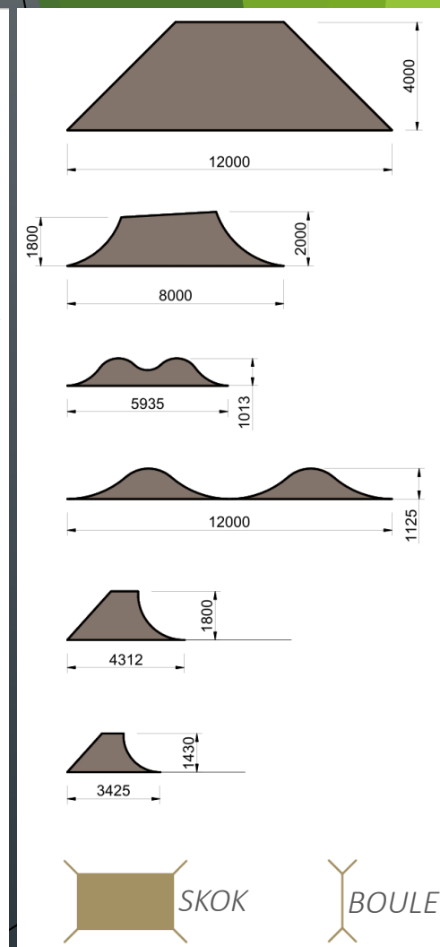
ŘEZ - PŘEKÁŽKY
